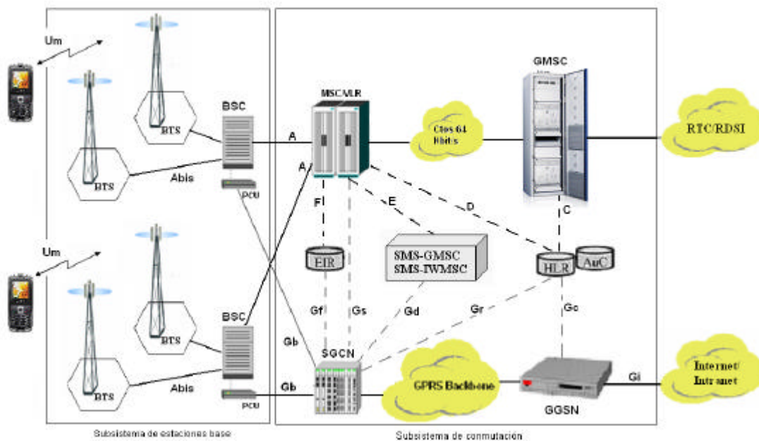
Figura 2.3 - Arquitectura básica de una red GSM/GPRS
