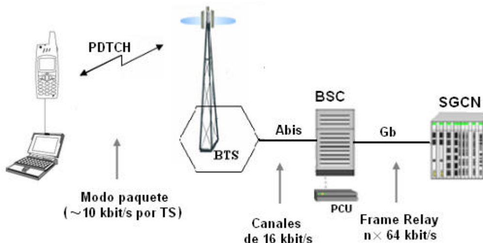
Figura 2.5 - Transporte de datos GPRS en la red de acceso
