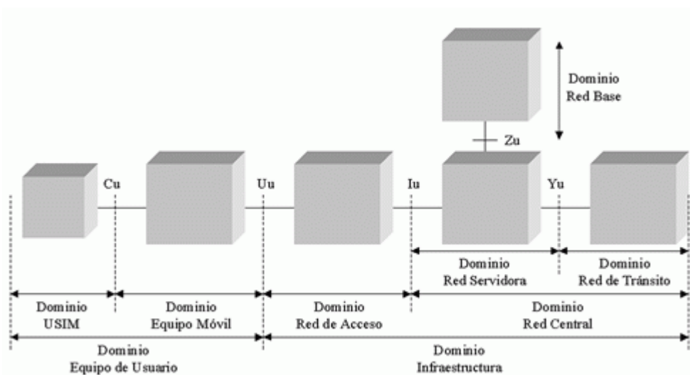
Figura 2.1 - Arquitectura general de un sistema UMTS
