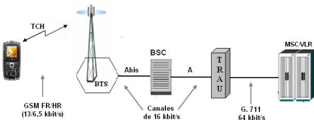
Figura 2.4 - Transporte de voz en la red de acceso GSM
