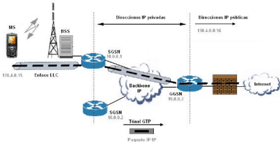
Figura 2.6 - Tunelado de datos sobre el “backbone” GPRS
